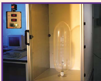
Teste de rutura para garantia de segurança
